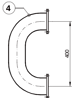
B N.2 CURVE DN 100 Flangia APAG DN 100
