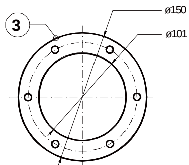
FLANGIA APAG DN 100
